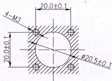
面板安装孔尺寸 Panel Size
